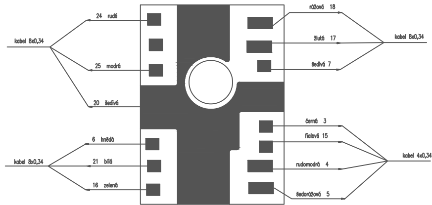
Připojení pájecí destičky (směr kabely do CAN 26)
