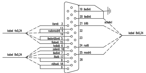
Zapojení CAN 26 vodiče do pistole (pohled pájení)
