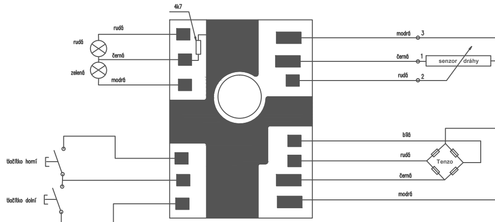
Připojení pájecí destičky (směr součástky v pistolí)
